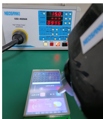
3.1 静电放电测试图 Electrostatic discharge test
