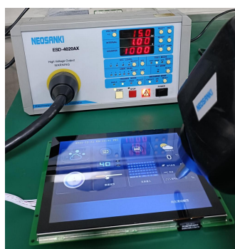
3.1 静电放电测试图
